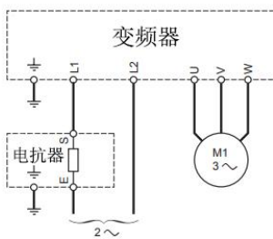
单相输入电抗器接线图
