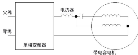
单相输出电抗器接线图
